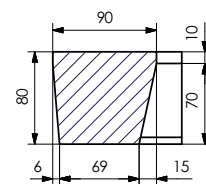
Secțiune B-B
