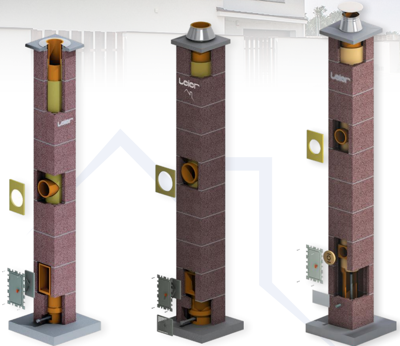
Sistemul de coș de fum Multikeram
